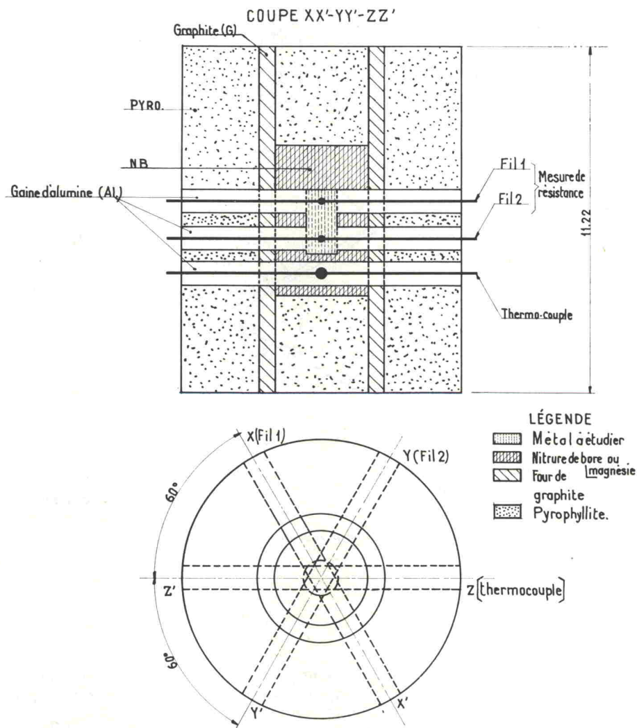
Fig. 5. — Cellule n° 2 pour mesure de résistivité en chauffage indirect sous haute pression (four cylindrique).
