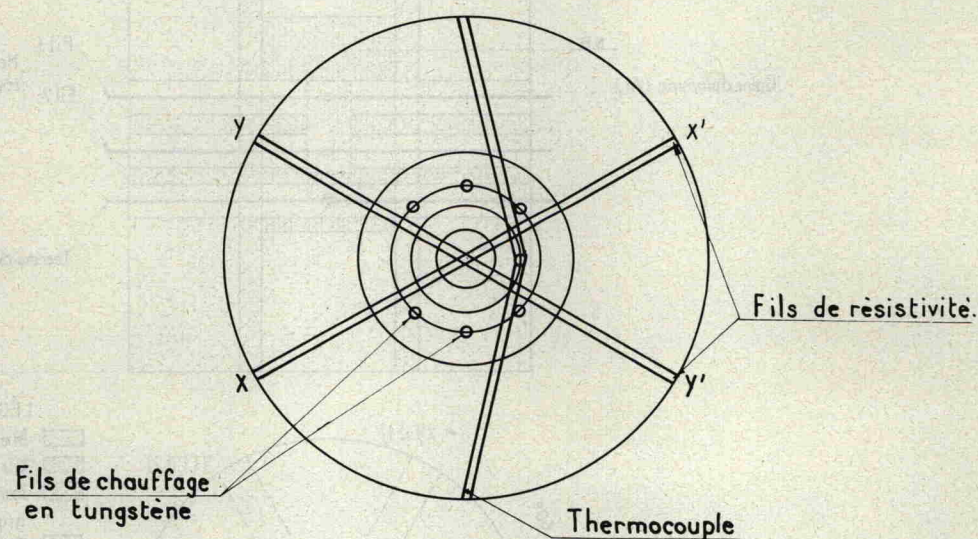
Fig. 6. — Cellule 2 bis, pour mesure de résistivité en chauffage indirect sous haute pression (four en cage).
